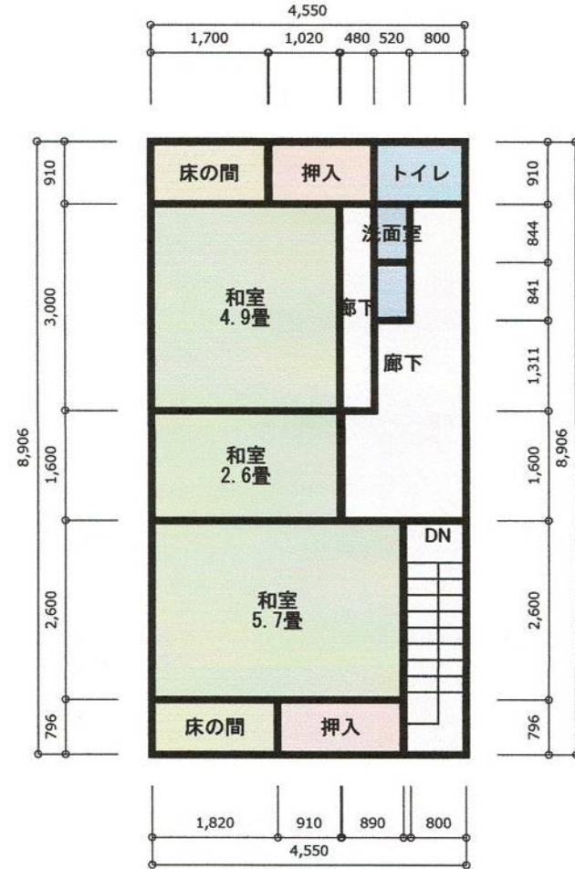
2階 縮尺 1/100
