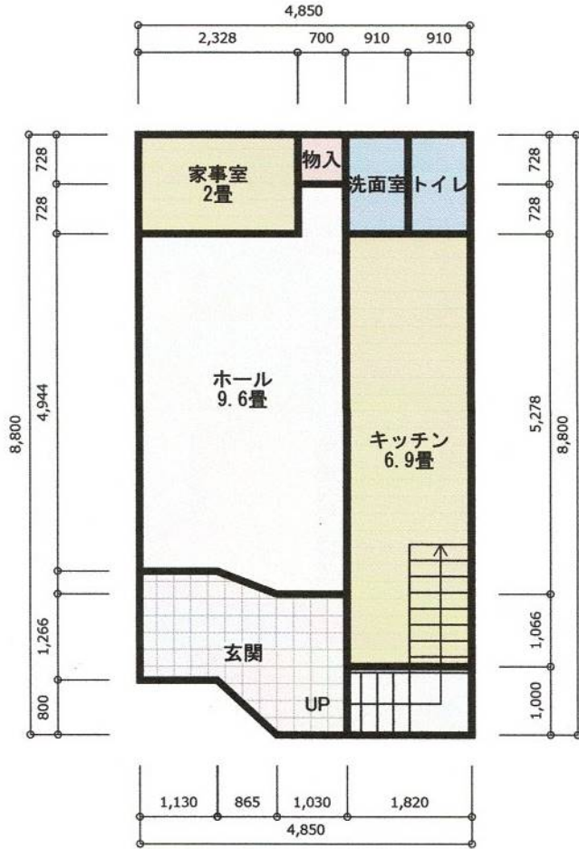
1階 縮尺 1/100
